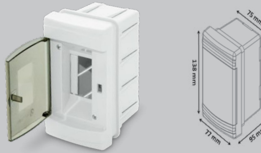
2'li Siva Altı Sigorta Kutusu 2 Module Distribution Box - Recessed
