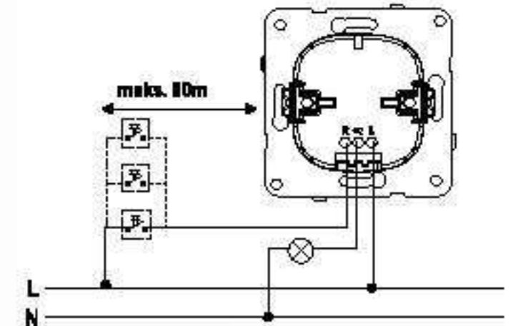
Light Anahtarı Çoklu Kullanımı
