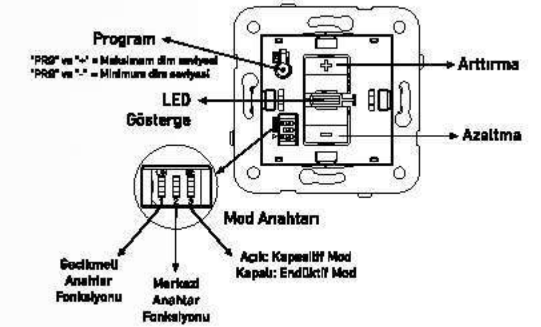
Merkezi Anahtar ile Kullanım
