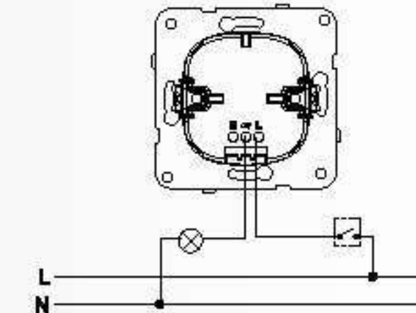
Merkezi Anahtar ile Kullanım
